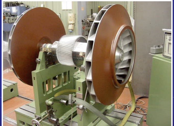
Demag VK Compressor Pinion
